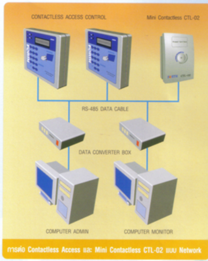
การต่อ Contactless Access กับ Mini Contactless CTL-02 แบบ Network
